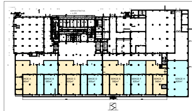
SITUACE 2.NP
