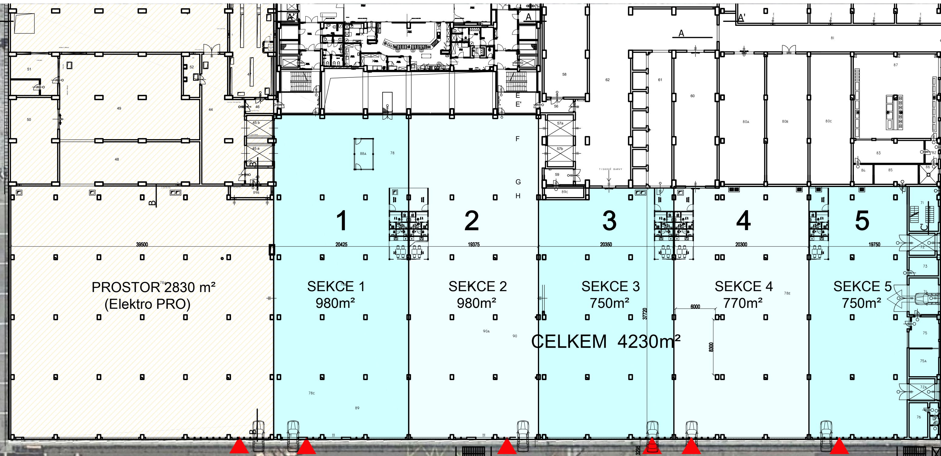
PŮDORYS 1.NP
